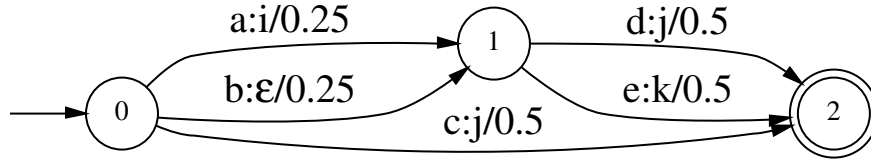
(a) T_{X,Y}
