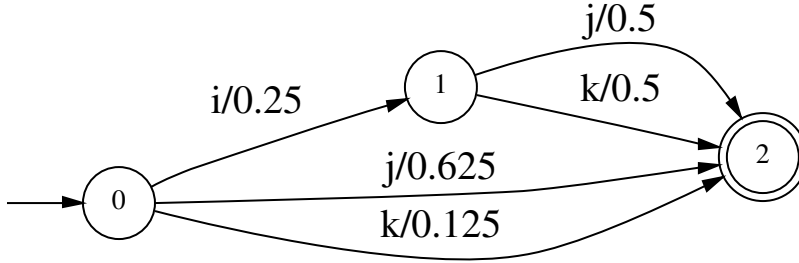
(b) T_Y
